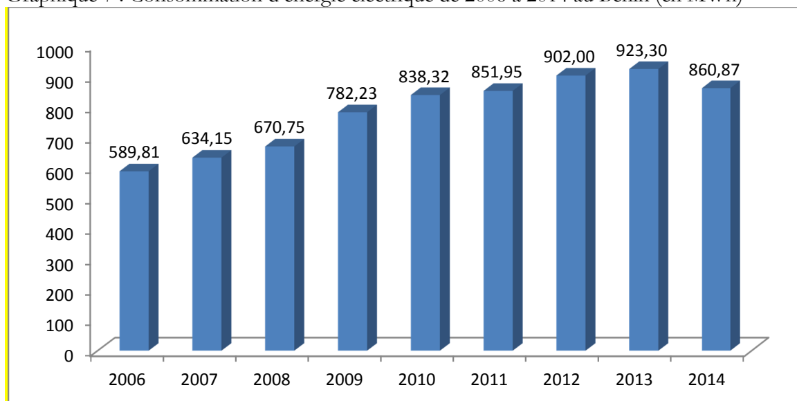
Graphique 7 : Consommation d'énergie électrique de 2006 à 2014 au Bénin (en MWh)
